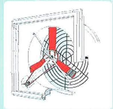
MF50C断面概略図
